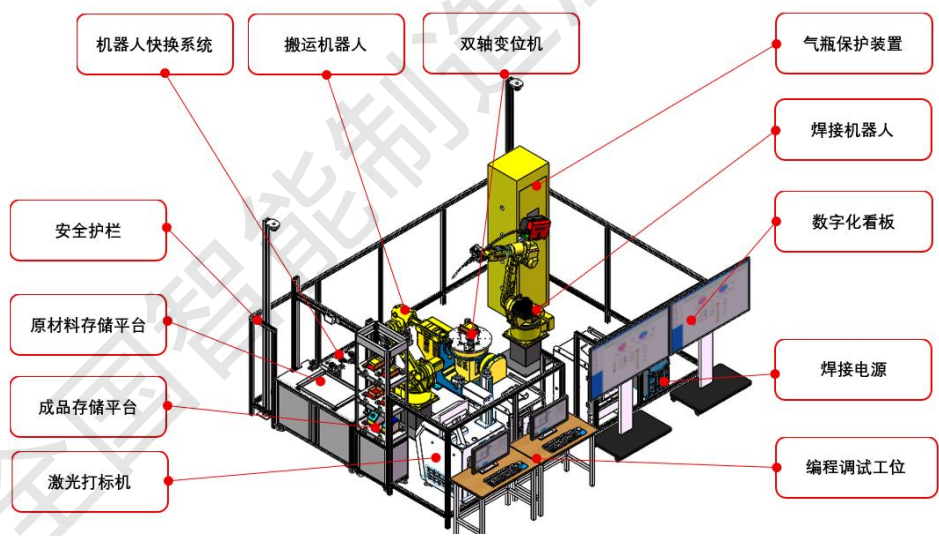
图 1 焊接设备装配调试工竞赛平台总布局简图
