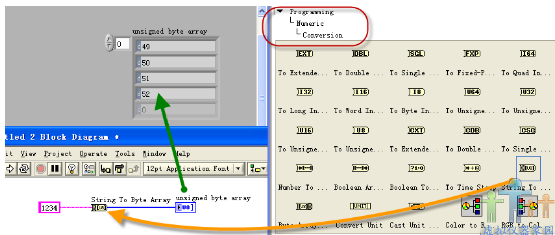
图 9 字符串转换为字节数组
