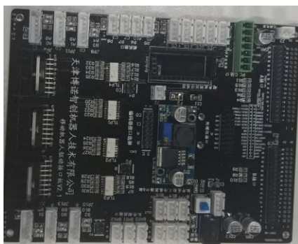
图 3 控制板实物图
