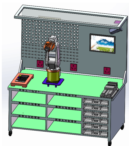
图4 拆装工作台
