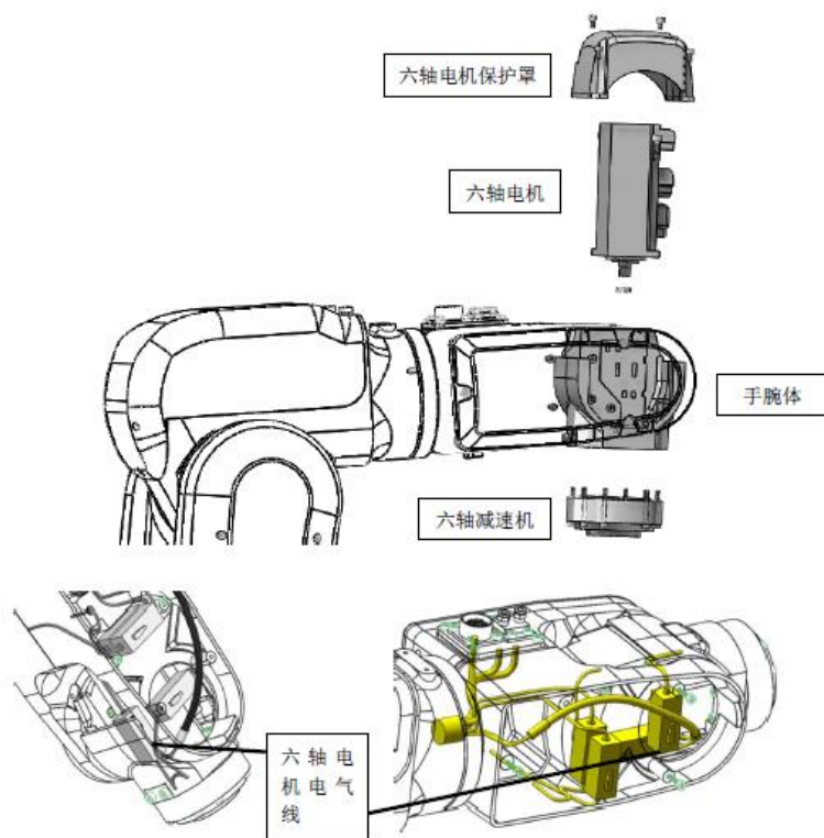
图 6 6 轴拆卸示意图
