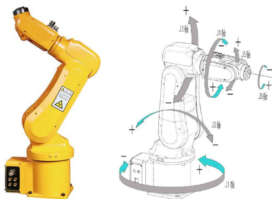
图5 6自由度工业机器人本体
